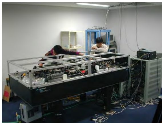
南極観測に用いたライダー送信系
