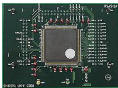
研究室で設計・試作した世界最速レベルの公開鍵暗号処理 LSI
